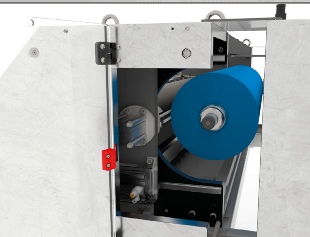
Cambio rapido della manica | Fast change of the sleeve
